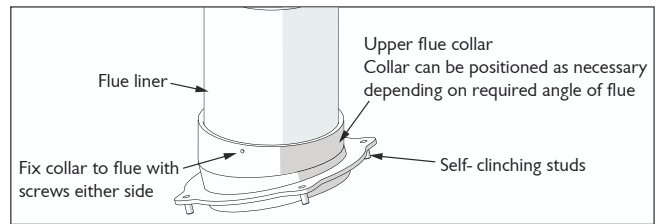
Fig. 13 Flue collar
